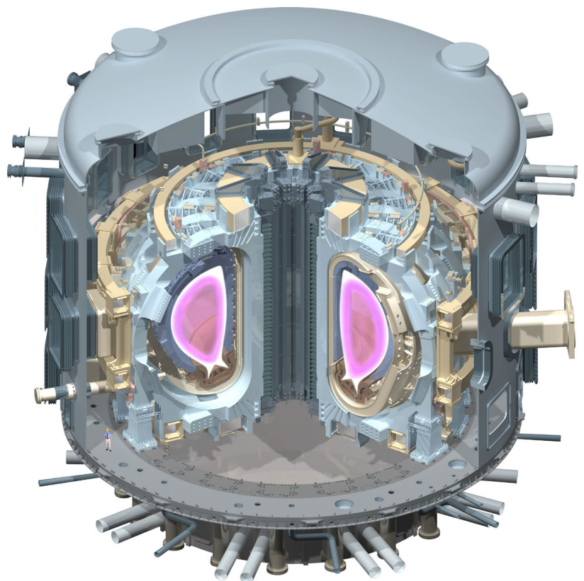
Der internationale Testreaktor ITER im Entwurf Grafik: ITER
